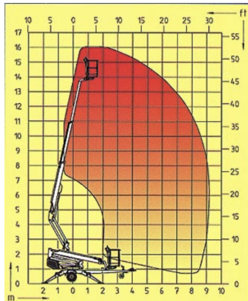
Arbeitsdiagramm:
