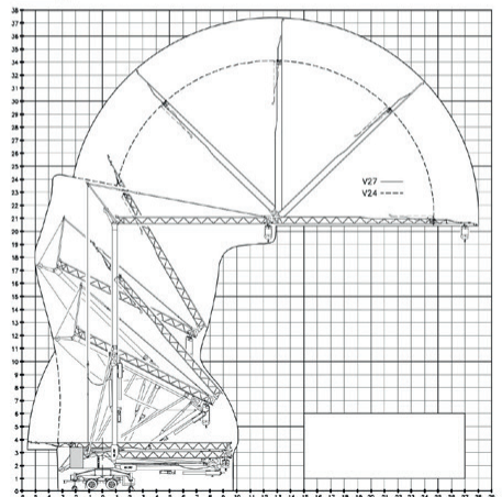
Montage
