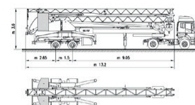
Montage
